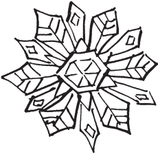
Spatial Dendrite
